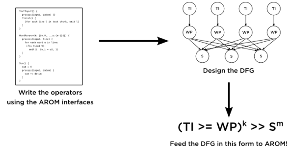
Figure 5 Définition d'un job dans AROM
